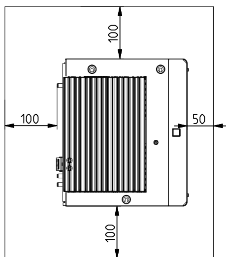
Abb. 1: Mindestabstände zu Begrenzungsflächen
