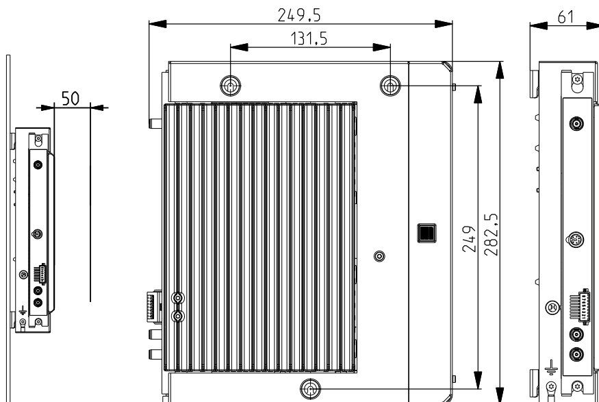
Abb. 2: Abmessungen und Montagepunkte
