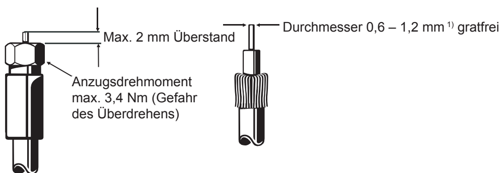
Abb. 3: Konfektionierung des F-Steckers
